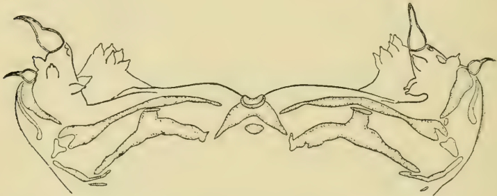
FIG. 32.— Lamippe papillifera Zulueta, ♀. Segundo par de patas. \times 565 .
